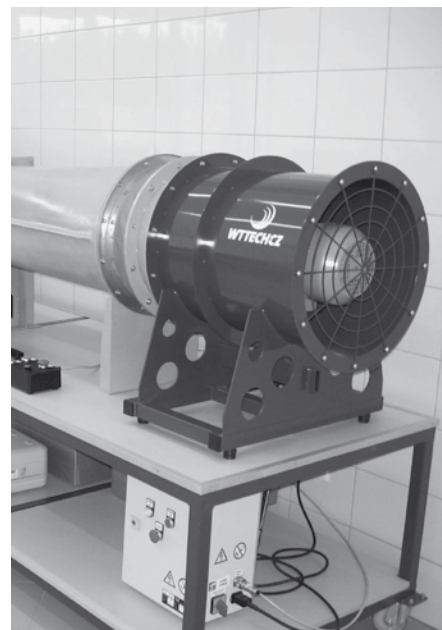
Tunel aerodynamiczny
